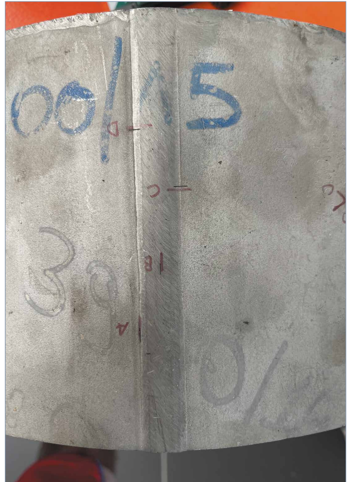
Realizzazione di intagli superficiali su saldatura in superduplex (dimensioni 5x2x0.2 mm).
