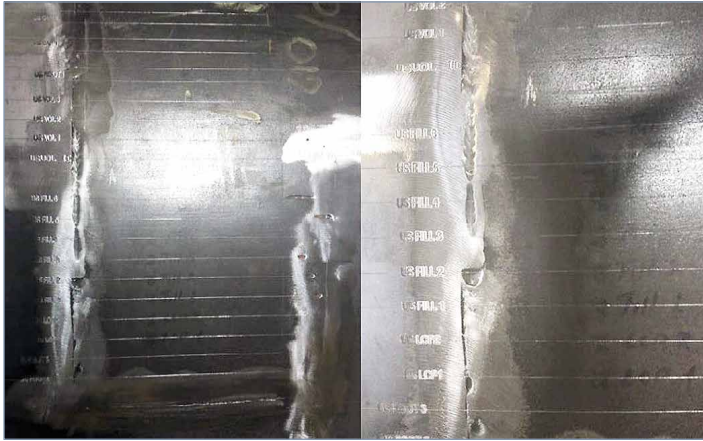
Blocco campione TOFD con saldatura testa-testa.
